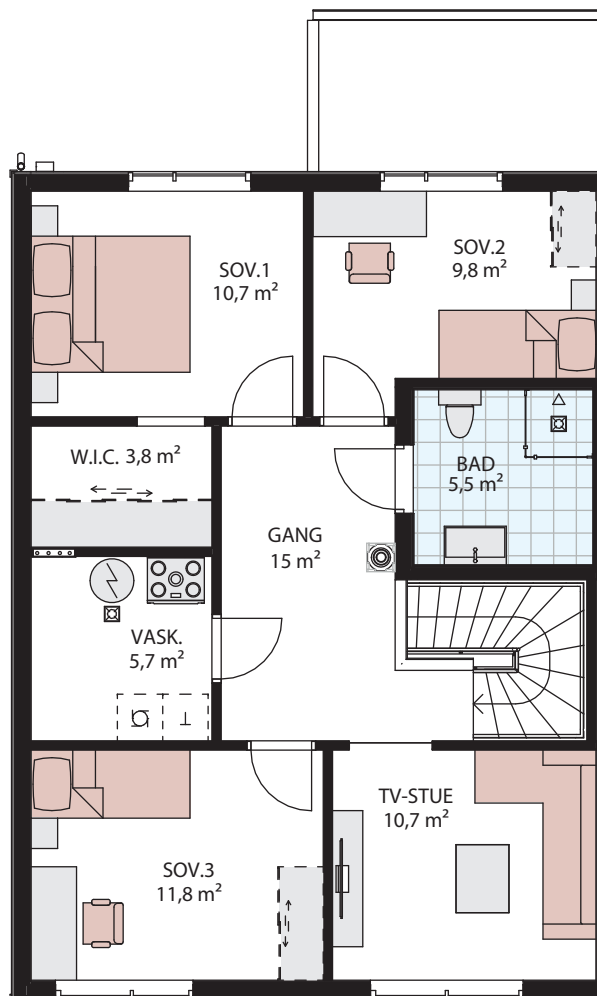
2. etasje
