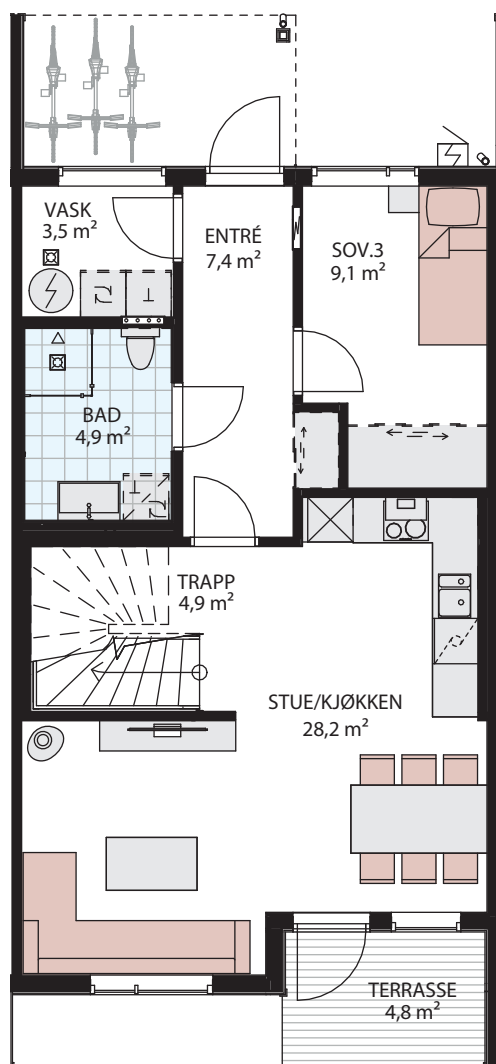
1. etasje
