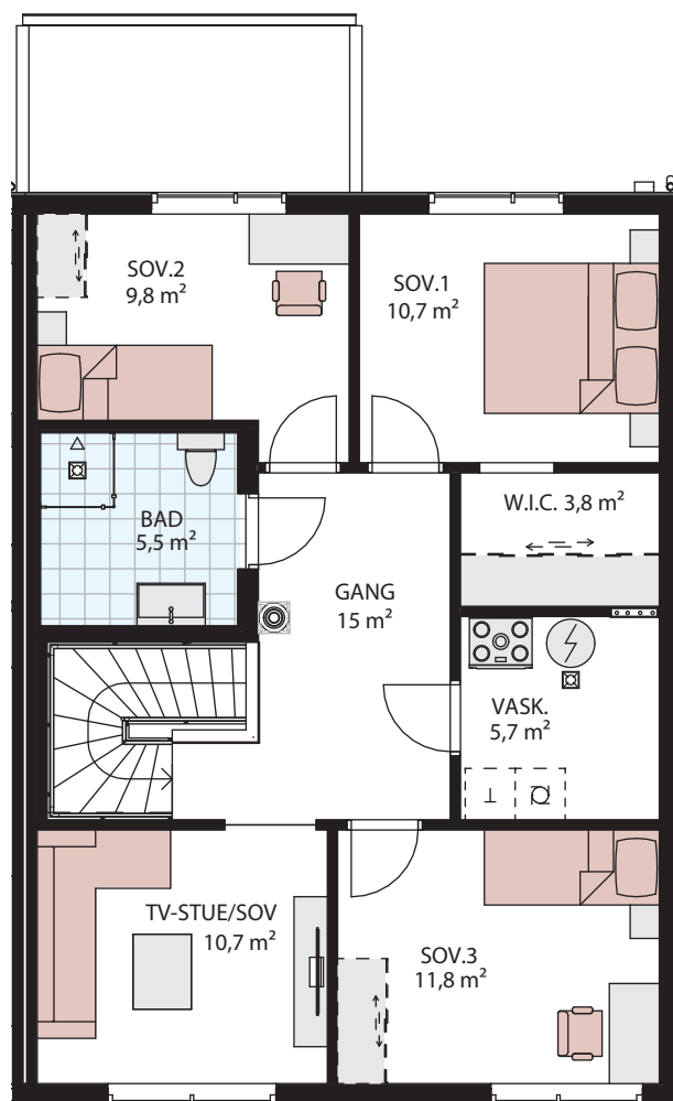
2. etasje
