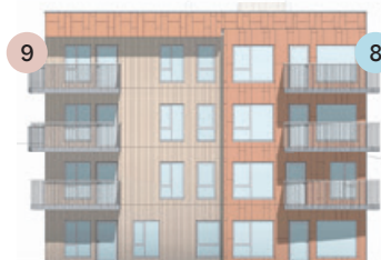
Fasade mot øst
