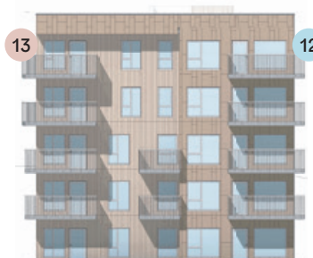
Fasade mot øst
