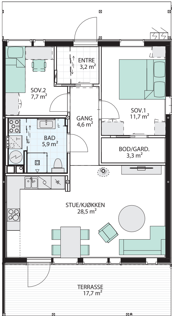
1. etasje Målestokk 1:100
