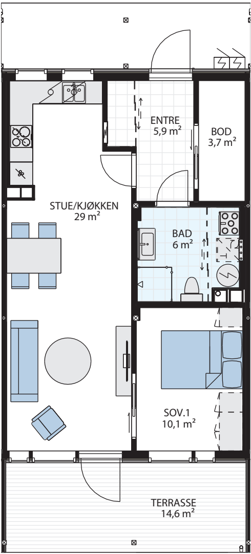
1. etasje Målestokk 1:100
