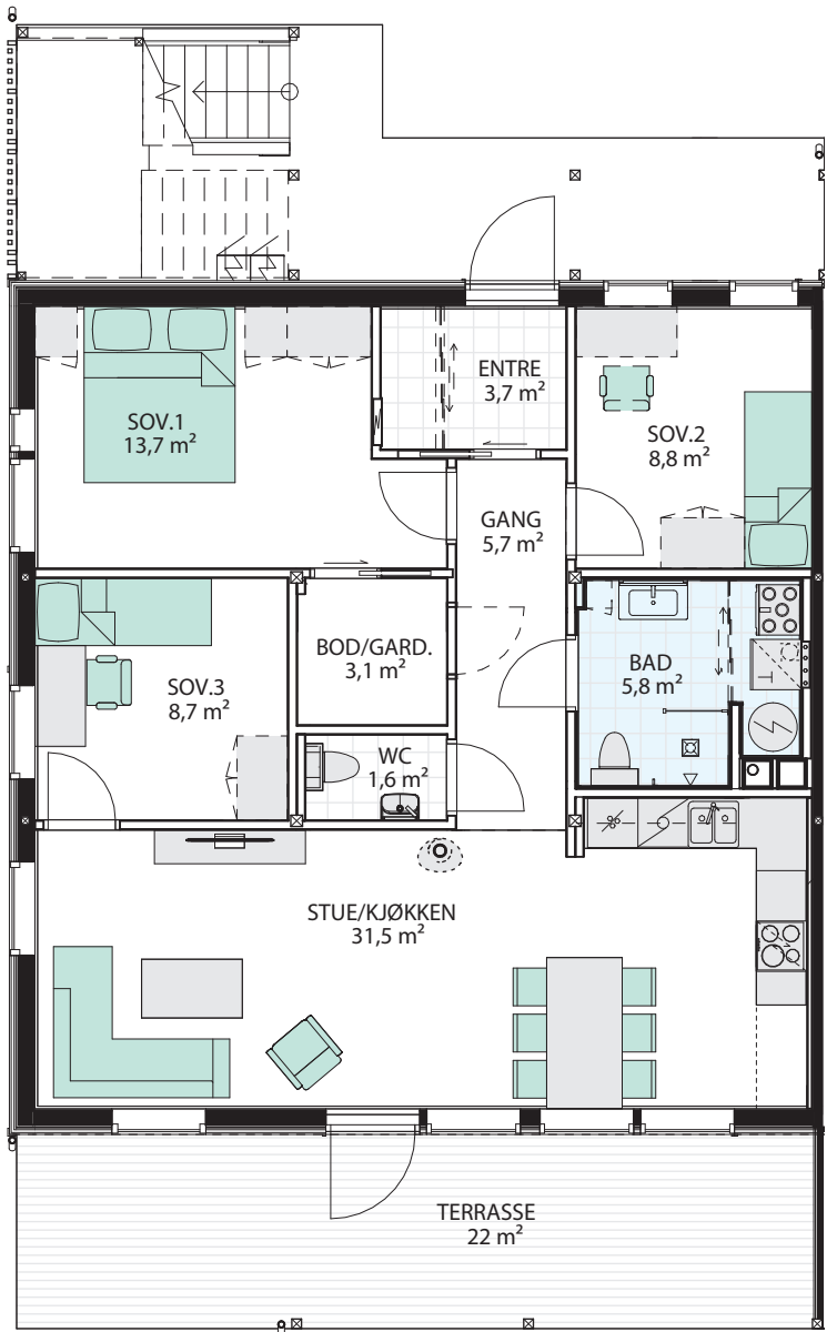
1. etasje Målestokk 1:100
